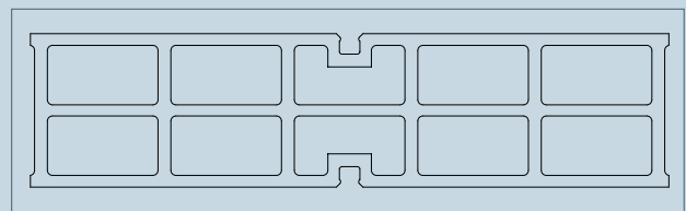
Draagstructuur van het rooster met een nominale breedte van 100 (500 x 123 mm)
