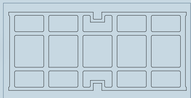
Draagstructuur van het rooster met een nominale breedte van 200 (500 x 223 mm)
