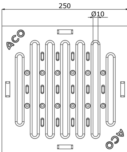
Grilles A 15 kN
