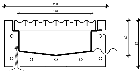
Technische doorsnede kanaal Modular 200.
